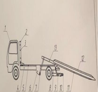
US20120195722 A1 Тасымалдау эвакуаторы Роберт Р. Нейлер
