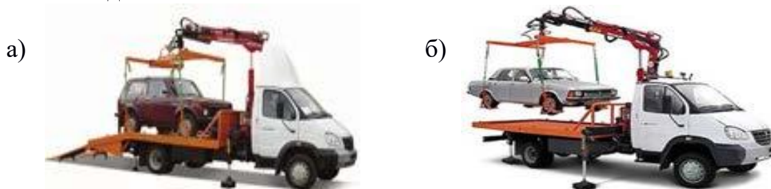
1.11- сурет- Гидроманипуляторы бар эвакуатор: а) - платформа көлбеу ; б) - түзу платформа
