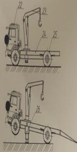
DE29805197 U1 Тасымалдау эвакуаторы Karlsson Theodor Klaus Gebri & Co KG
